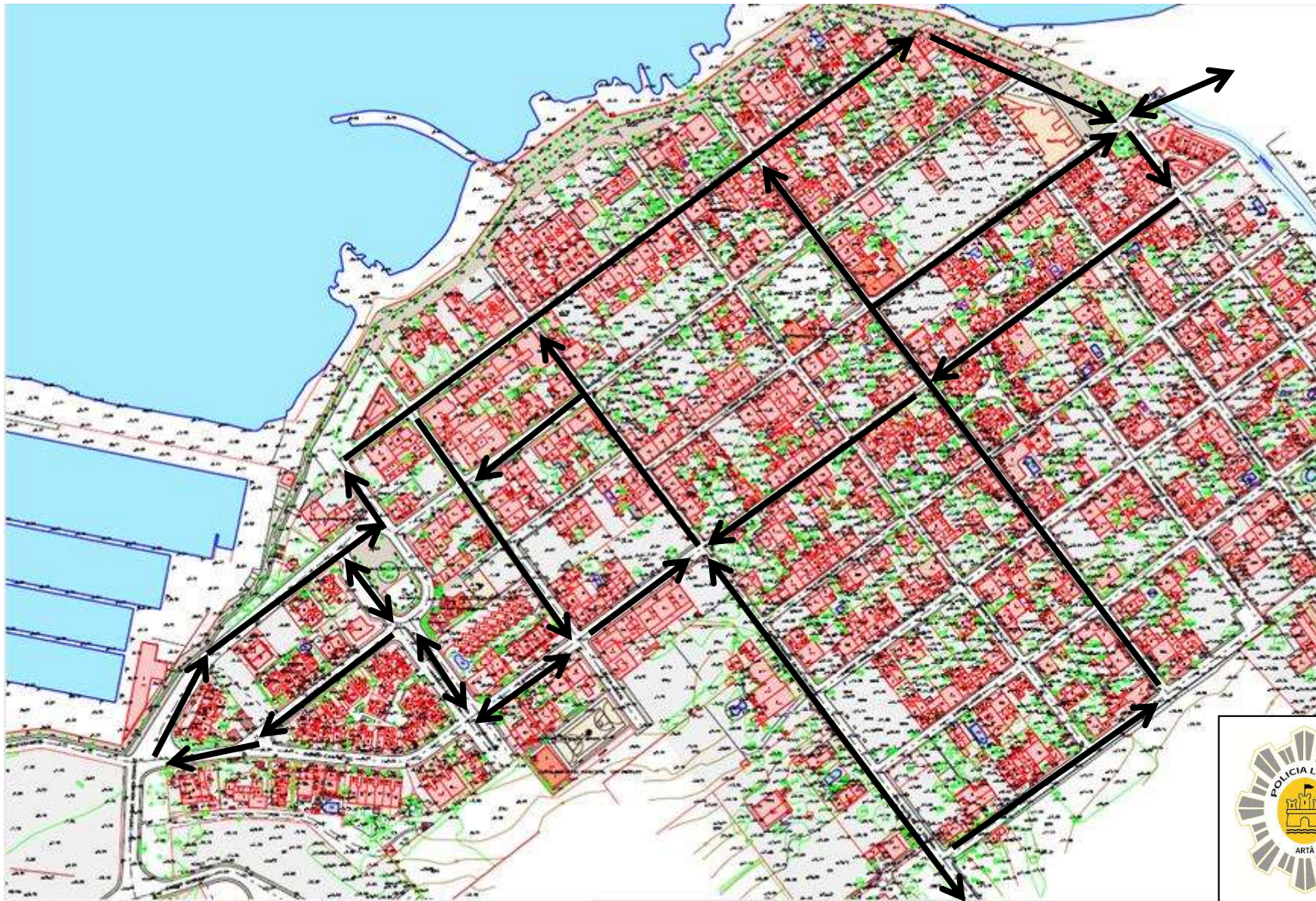
VIES D'ACCÉS I D'EVACUACIÓ PROGRAMADES PER ALS FOGUERONS SANT ANTONI- COLÒNIA DE SANT PERE
